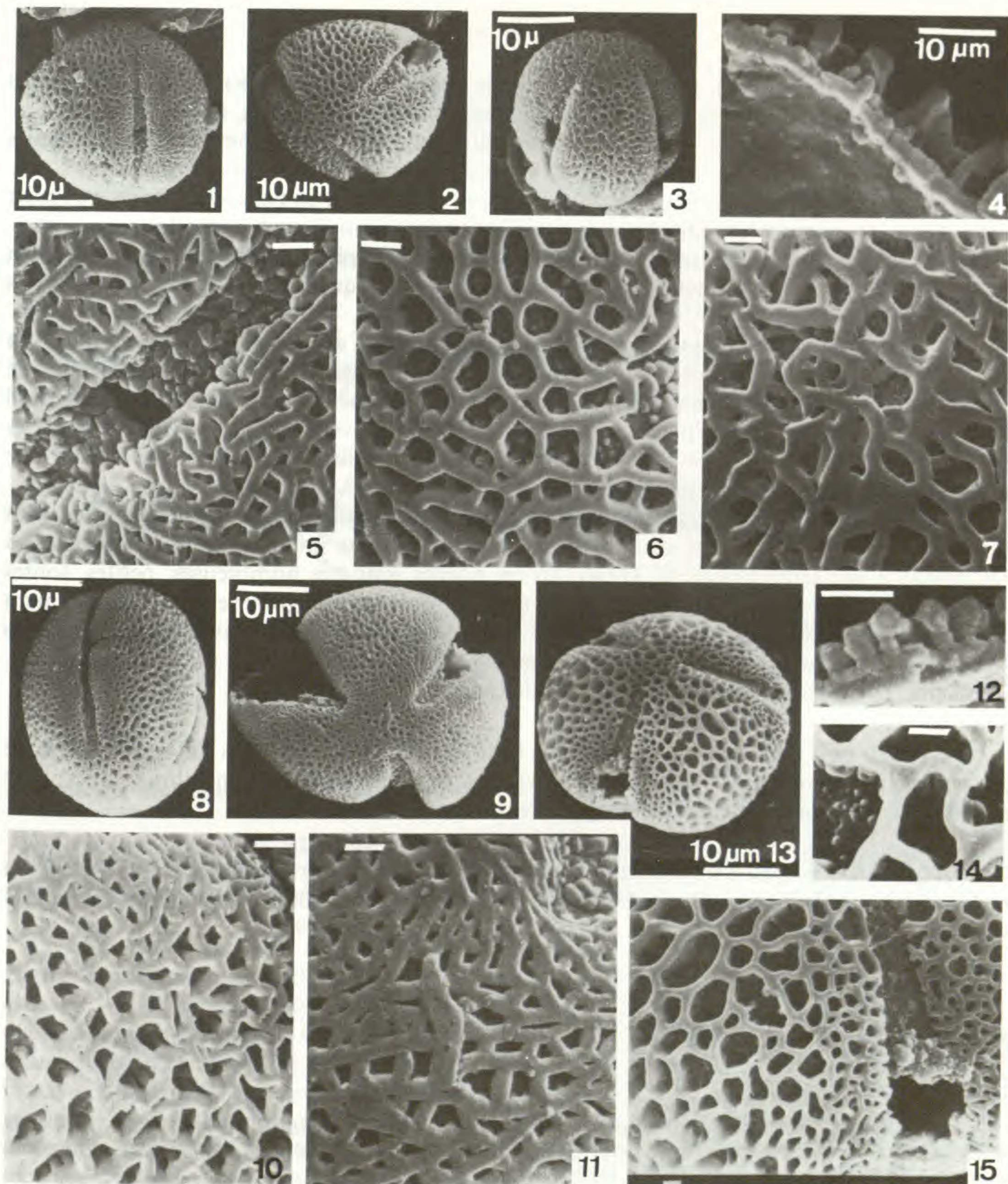
Fig. 2. — Pollens de Ptaeroxylaceae : Ptaeroxylon obliquum (Thunb.) Radlk. ( Story s.n. , P) : 1, aperture composée de face, marge diffuse peu marquée et légèrement rugulo-réticulée, membrane aperturale finement et régulièrement granuleuse ; 2, vue polaire ; 3, intercolpium ; 4, cassure montrant la structure de l'exine ; 5, membrane aperturale et marge diffuse ; 6, détail du réseau au pôle, verrues dans le fond des mailles ; 7, réseau à mailles irrégulières dans l'intercolpium. — Cedrelopsis grevei Baillon ( Capuron SF 29022 , P) : 8, marge à la limite tectée perforée — finement réticulée ; 9, vue polaire d'un grain à marge rugulo-réticulée ; 10, exine dans un intercolpium ; 11, détail de la vue polaire d'un grain à marge rugulo-réticulée ; 12, structure de l'exine. — C. trivalvis J.-F. Leroy ( SF 7698 , P) : 13, vue polaire oblique ; 14, verrues dans les mailles ; 15, marge réticulée, verrues dans les mailles. (Le trait d'échelle correspond à 1 \mu\text{m} , sauf indication).
